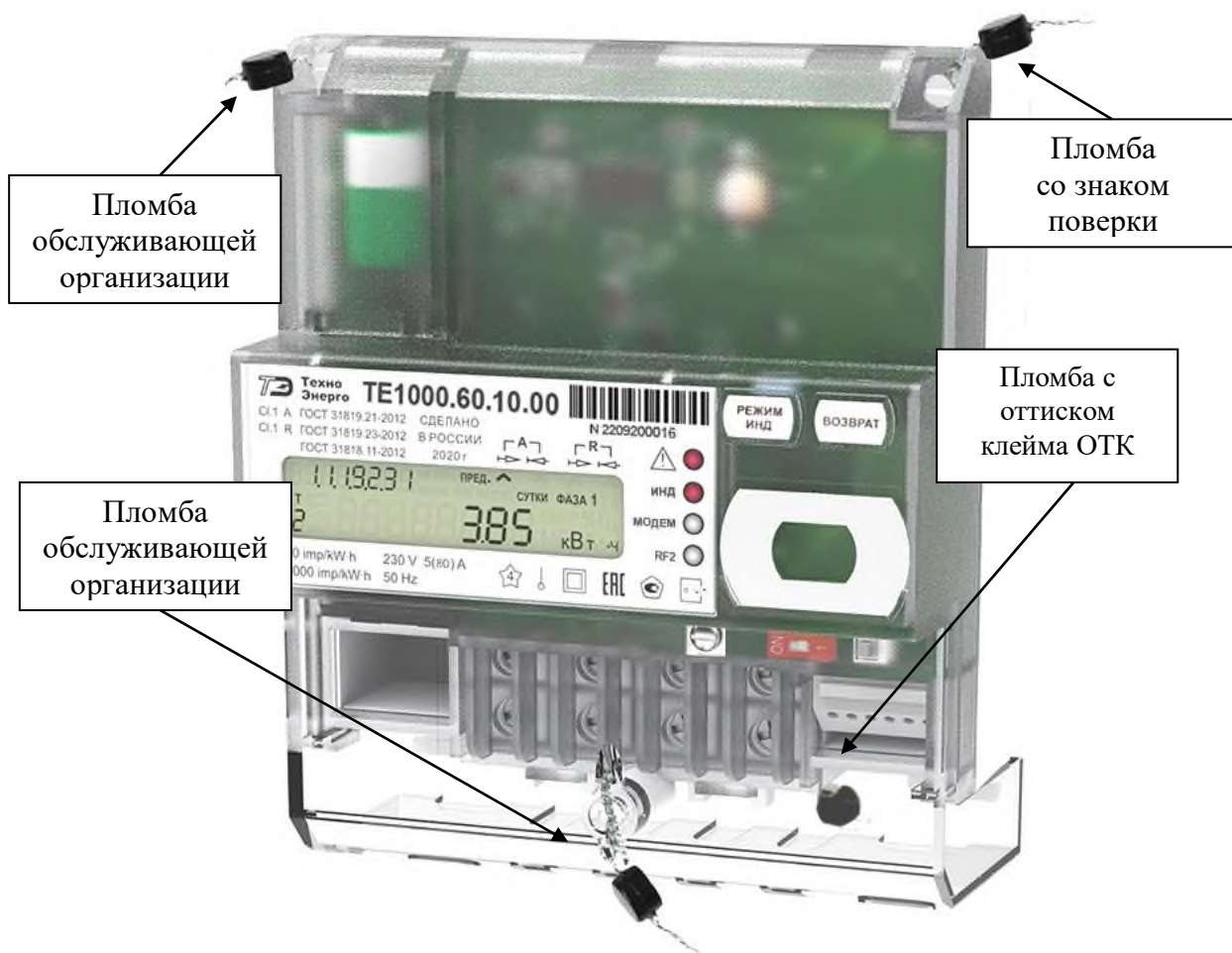
Рисунок 2 – Общий вид счетчика для установки на DIN-рейку, схема пломбировки от несанкционированного доступа, обозначение места нанесения знака поверки
